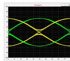
MSK eyes diagram
