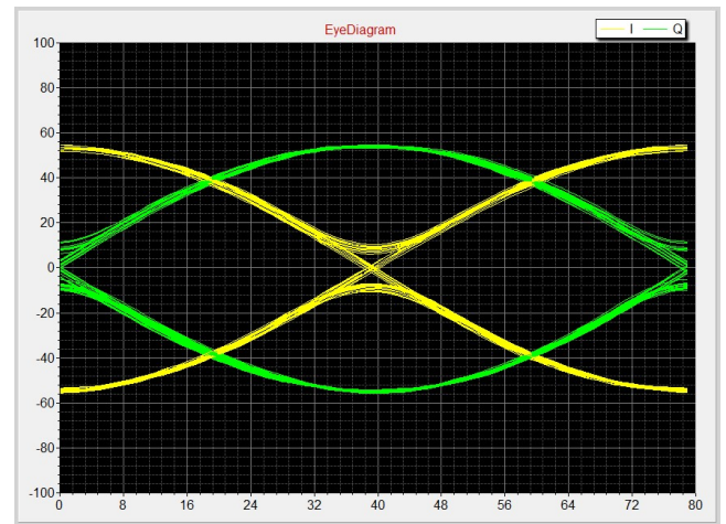
MSK eyes diagram
